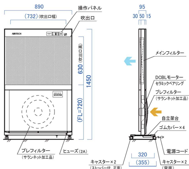
ACP-898LAH (装置背面吸込み)
