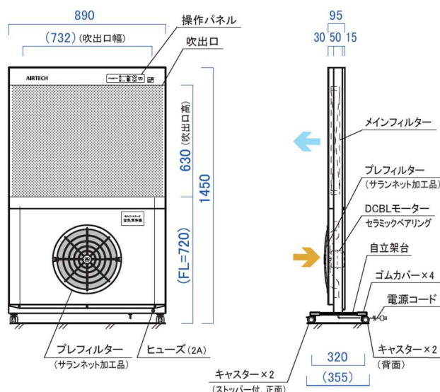
ACP-898LBH (装置前面吸込み)
