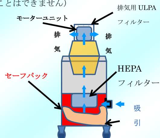
内蔵 HEPA フィルター
