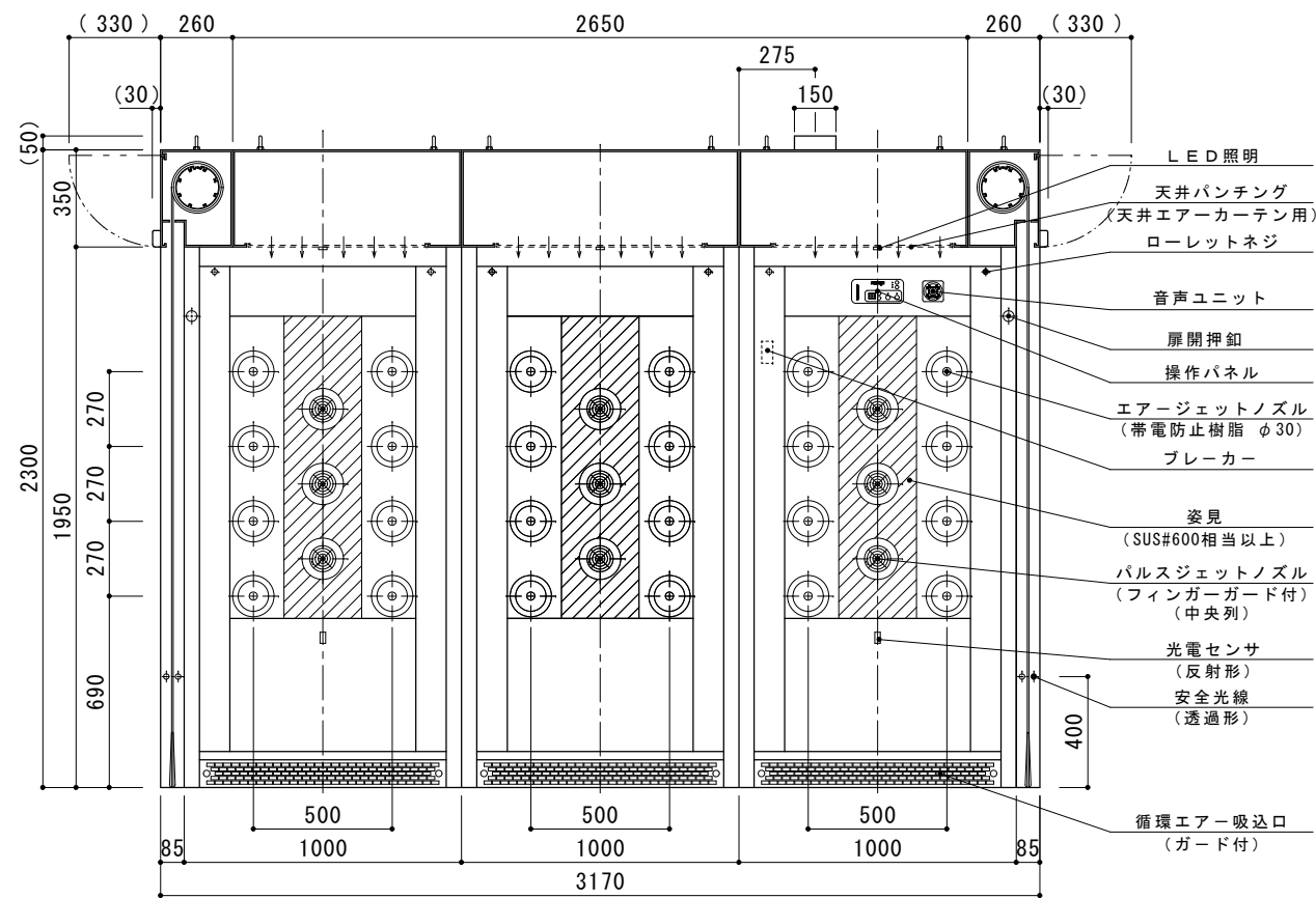
A-A' 断面
