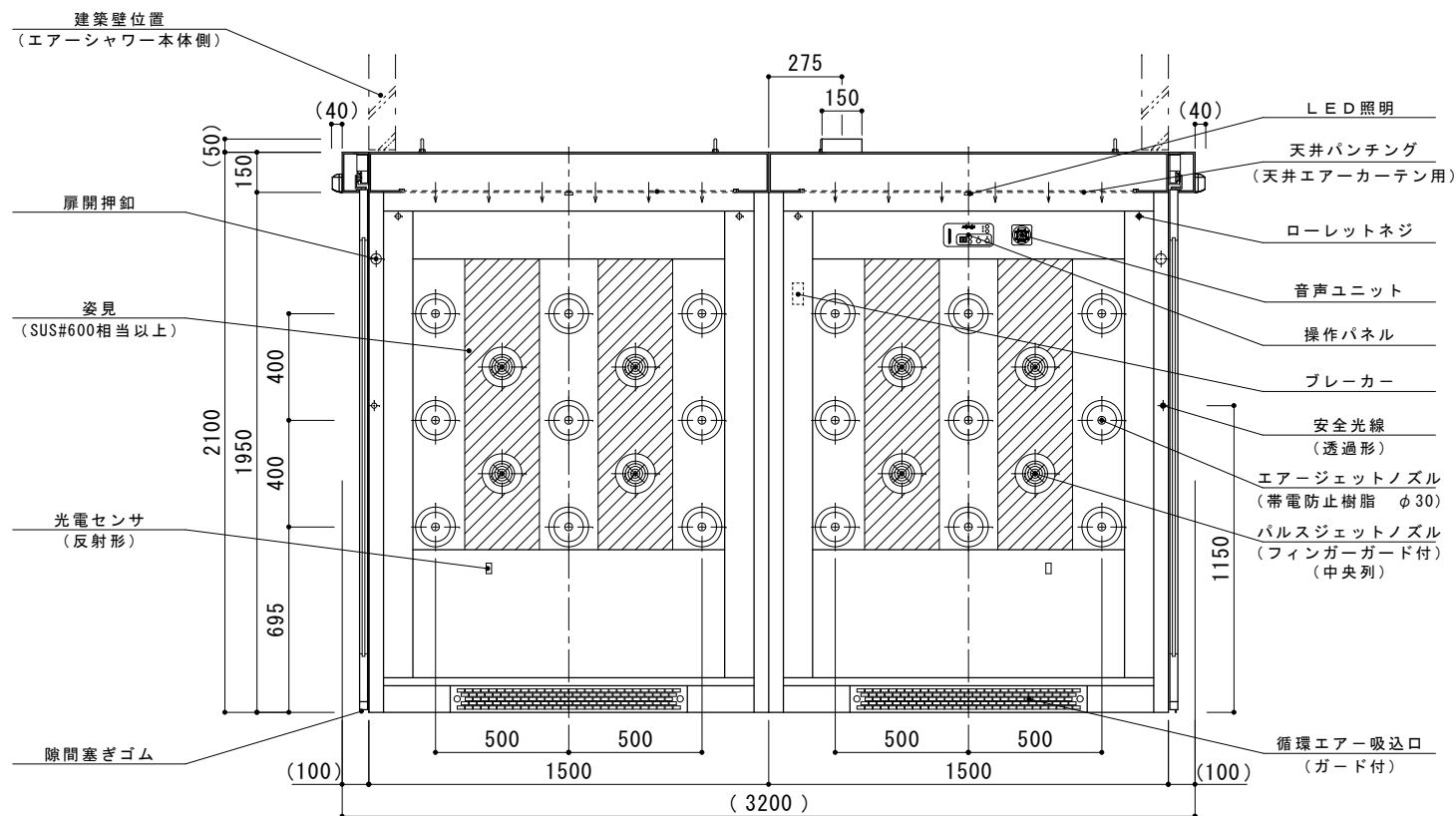
A-A' 断面
