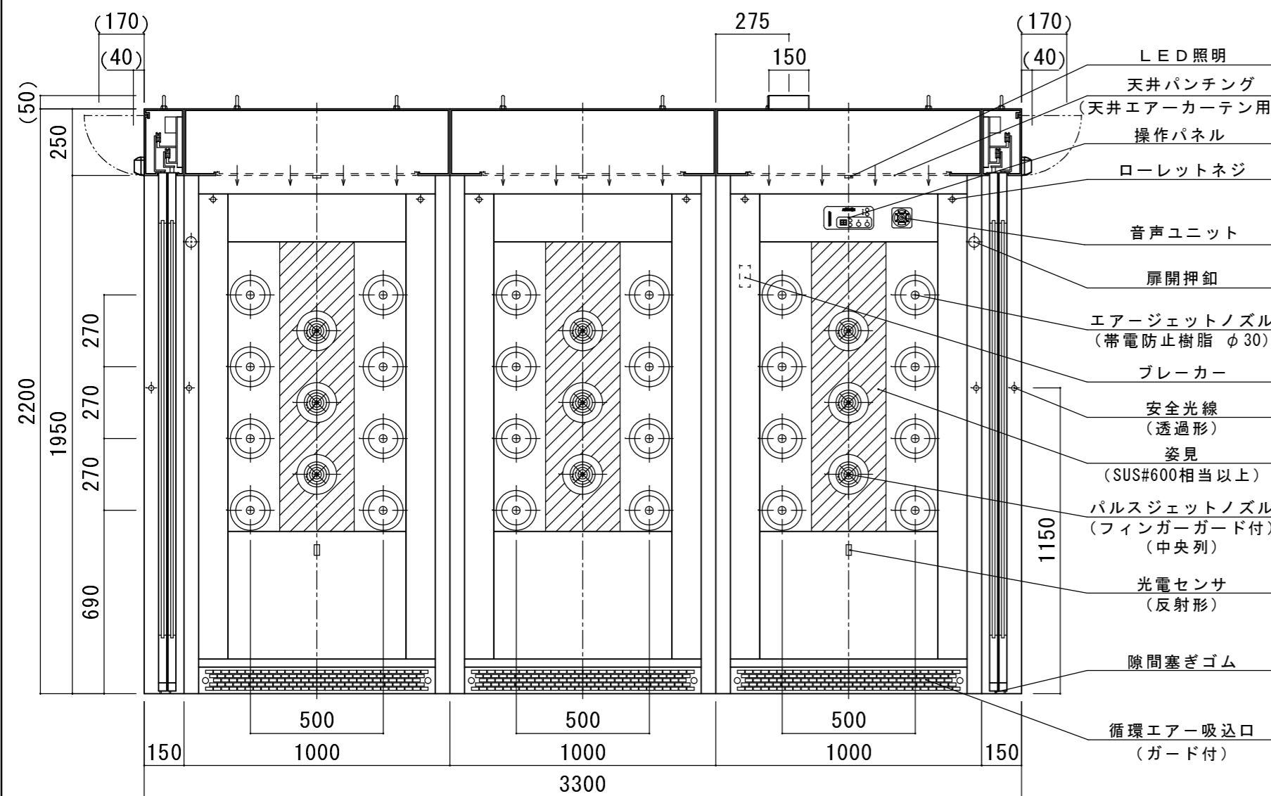
A-A' 断面
