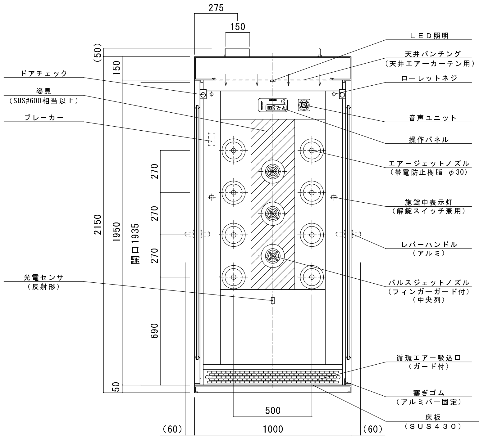
A-A'断面
