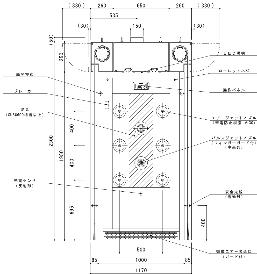
A-A' 断面
