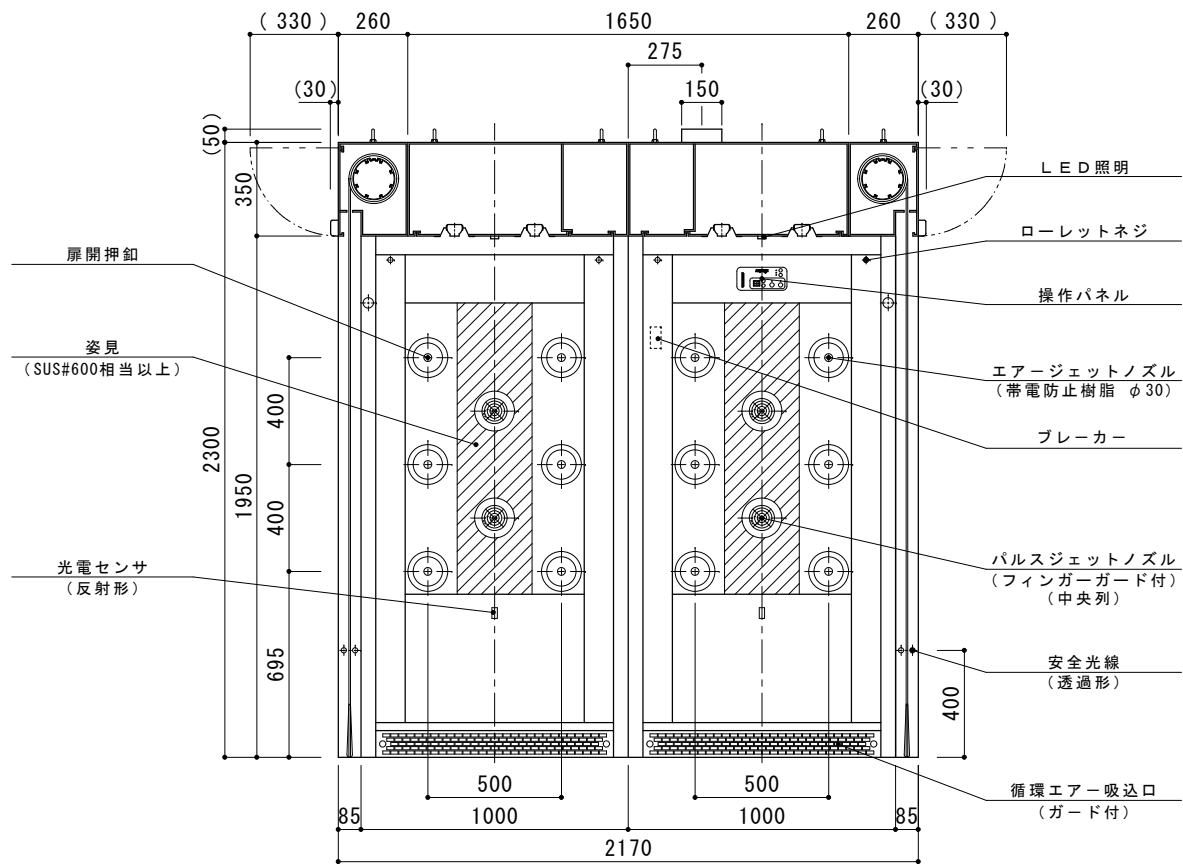
A-A' 断面
