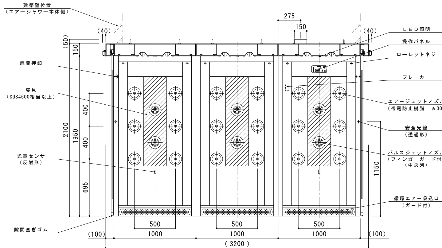
A-A' 断面
