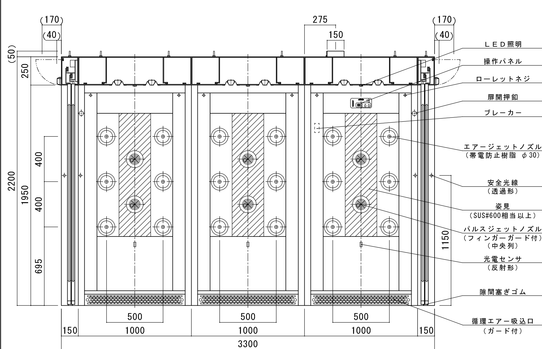
A-A' 断面
