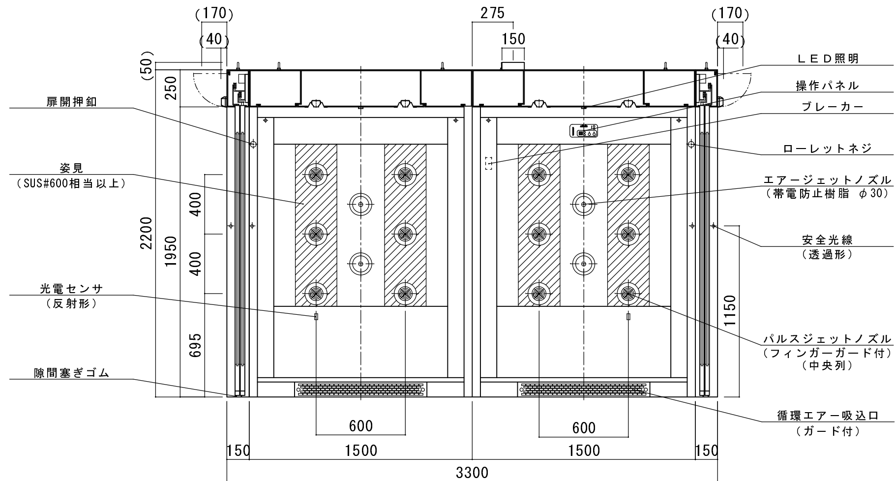
A-A' 断面
