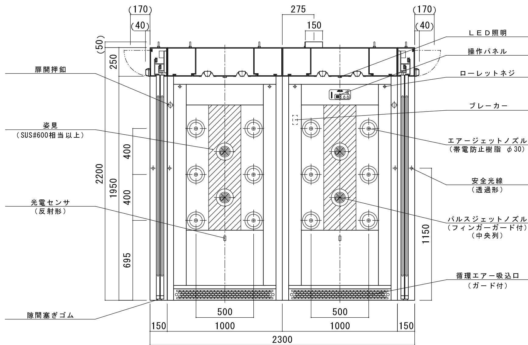
A-A' 断面
