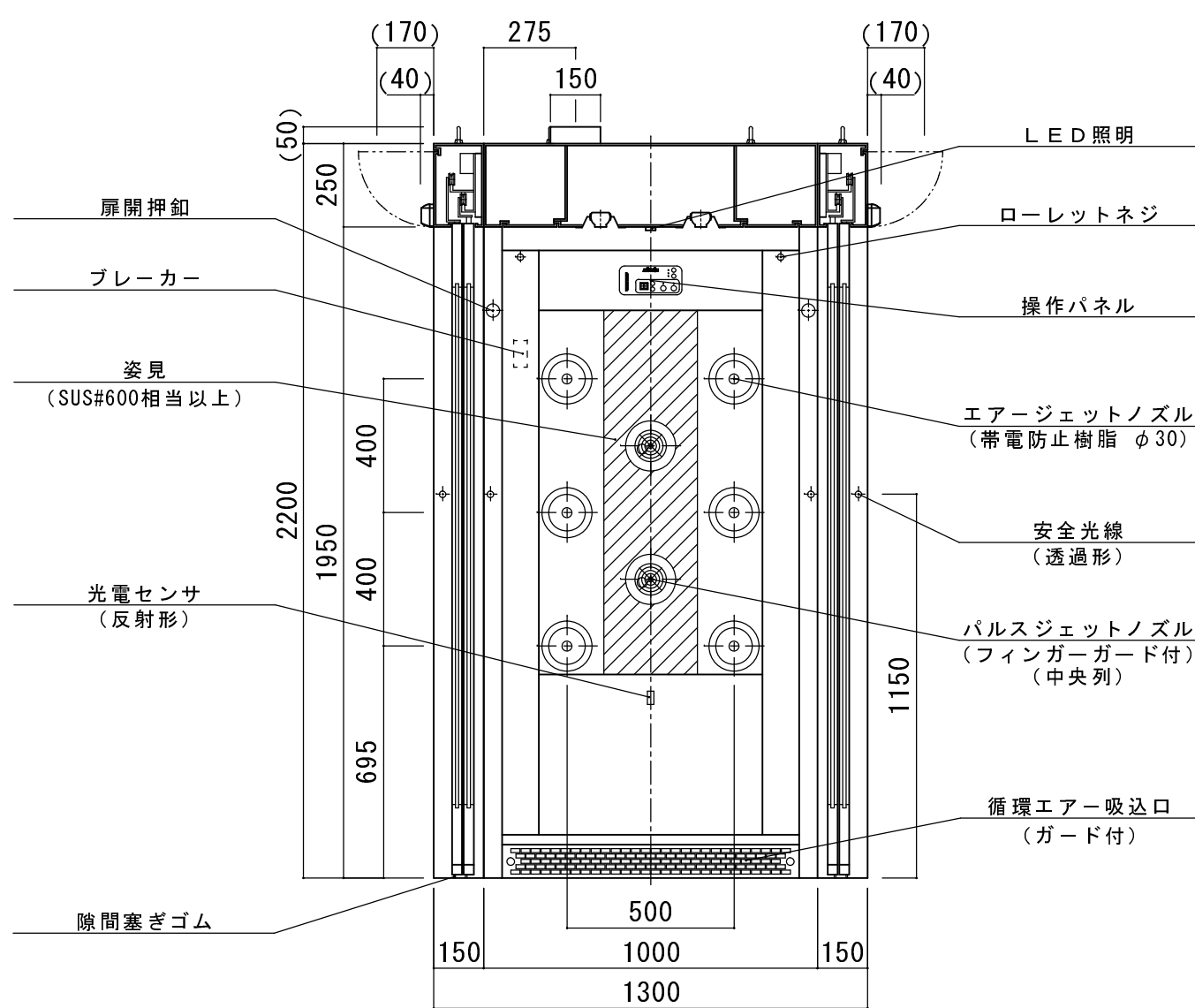
A-A' 断面
