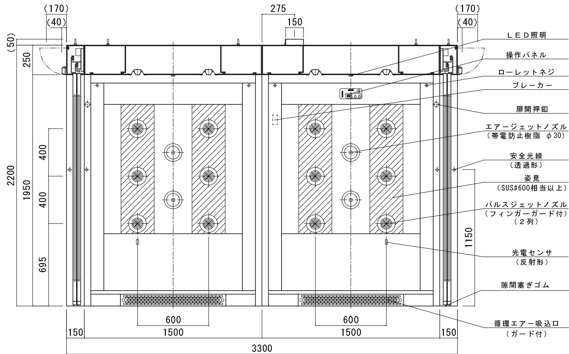
A-A' 断面
