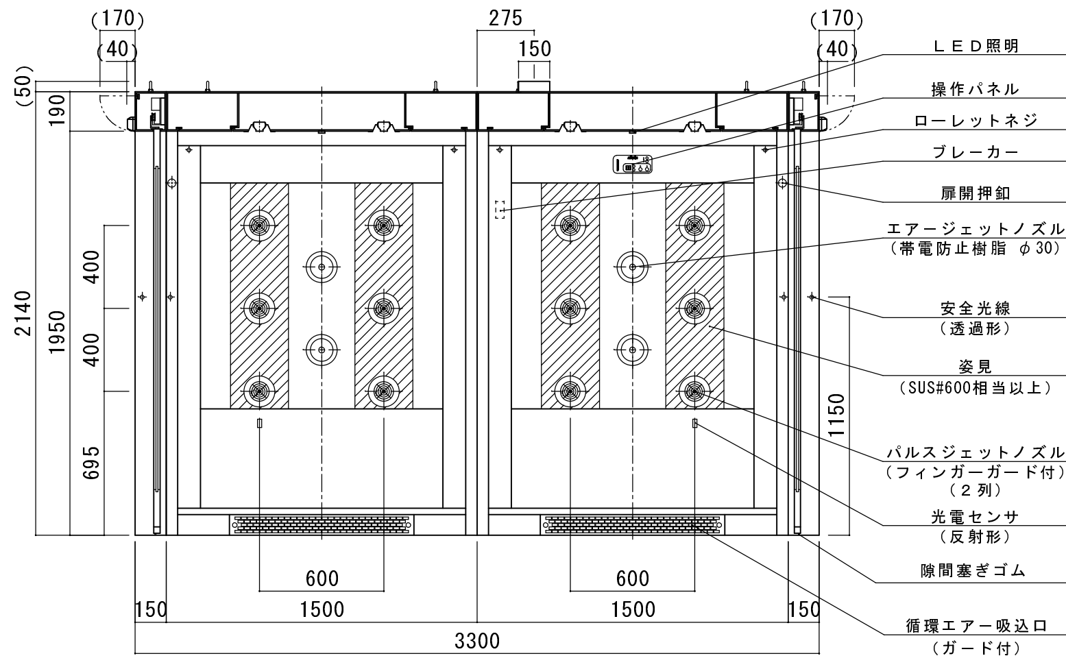
A-A' 断面
