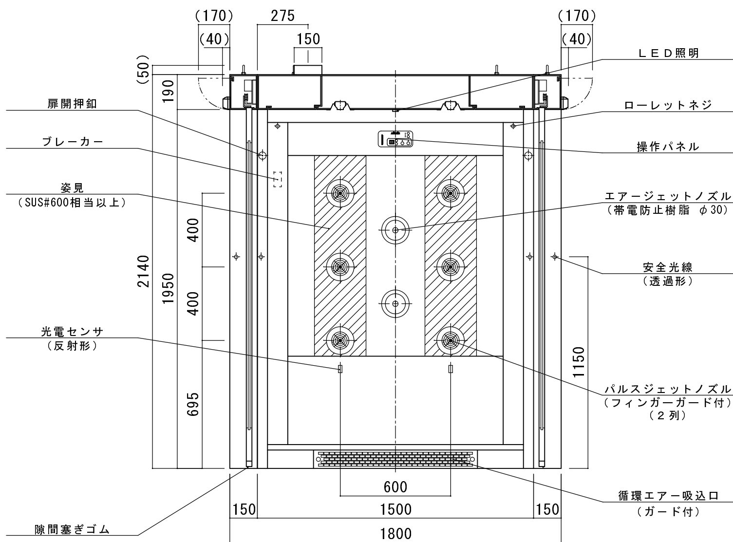
A-A'断面
