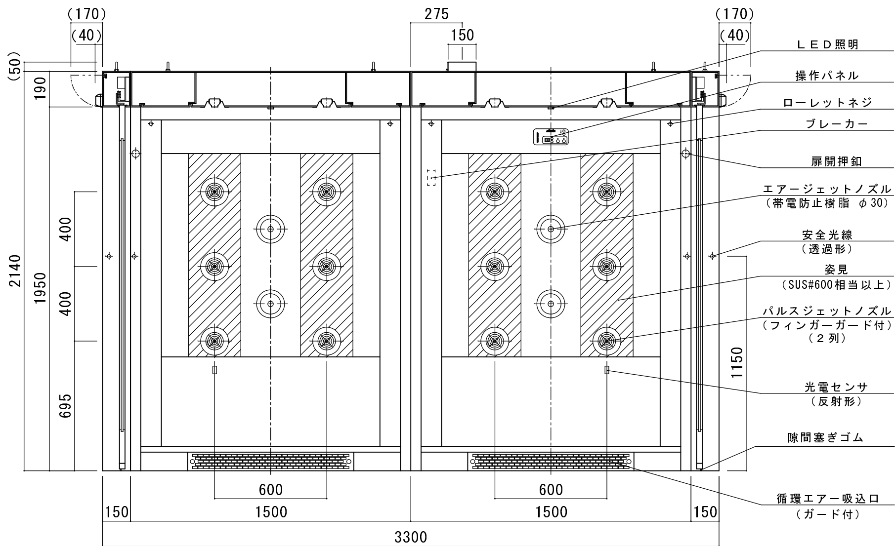
A-A' 断面
