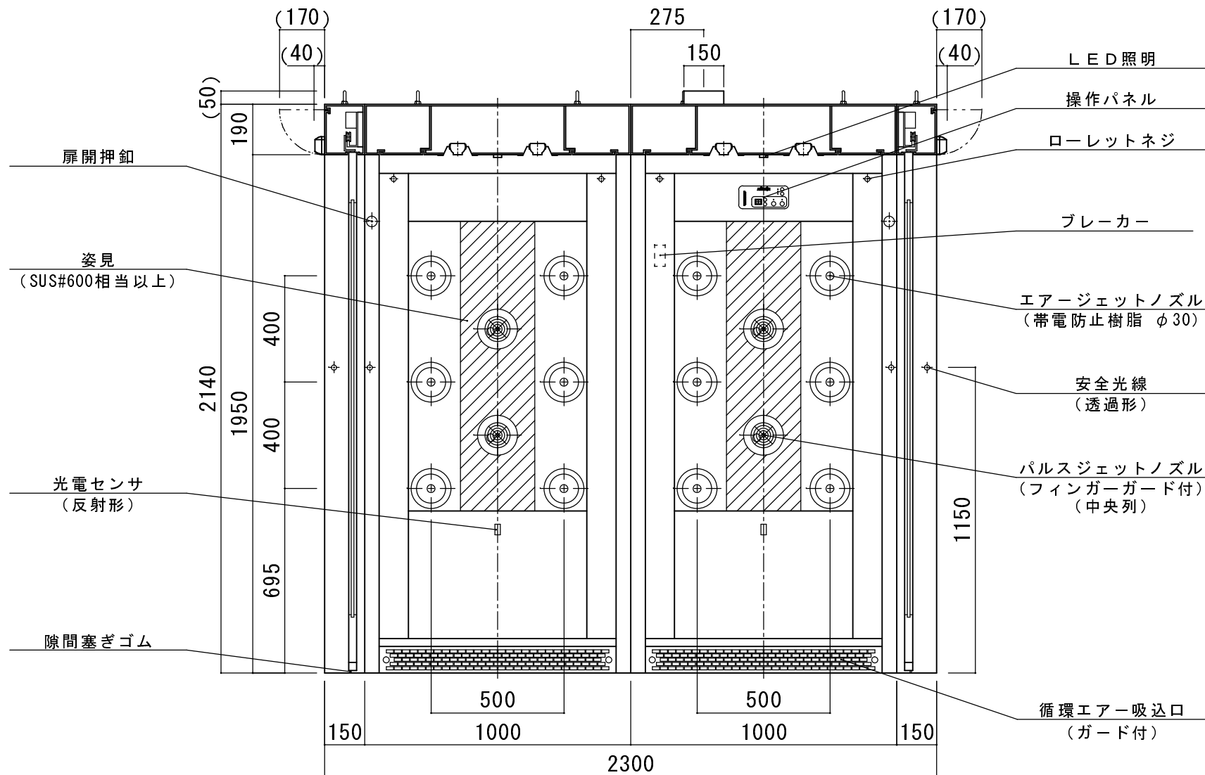
A-A' 断面
