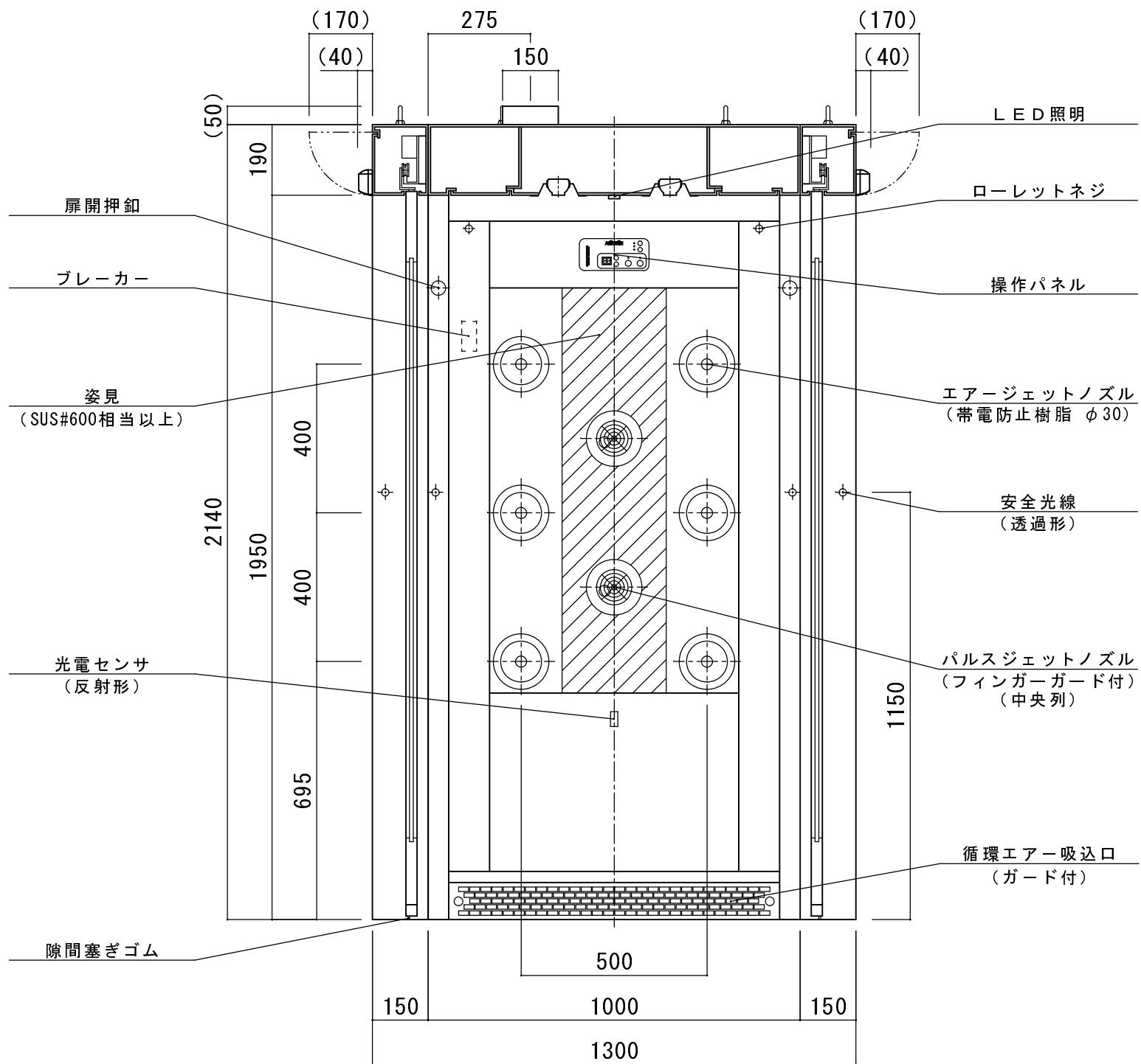
A-A' 断面
