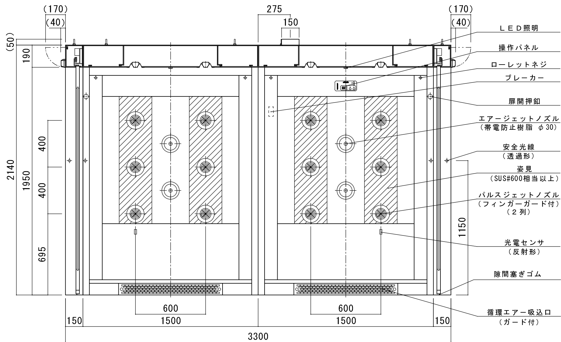
A-A' 断面
