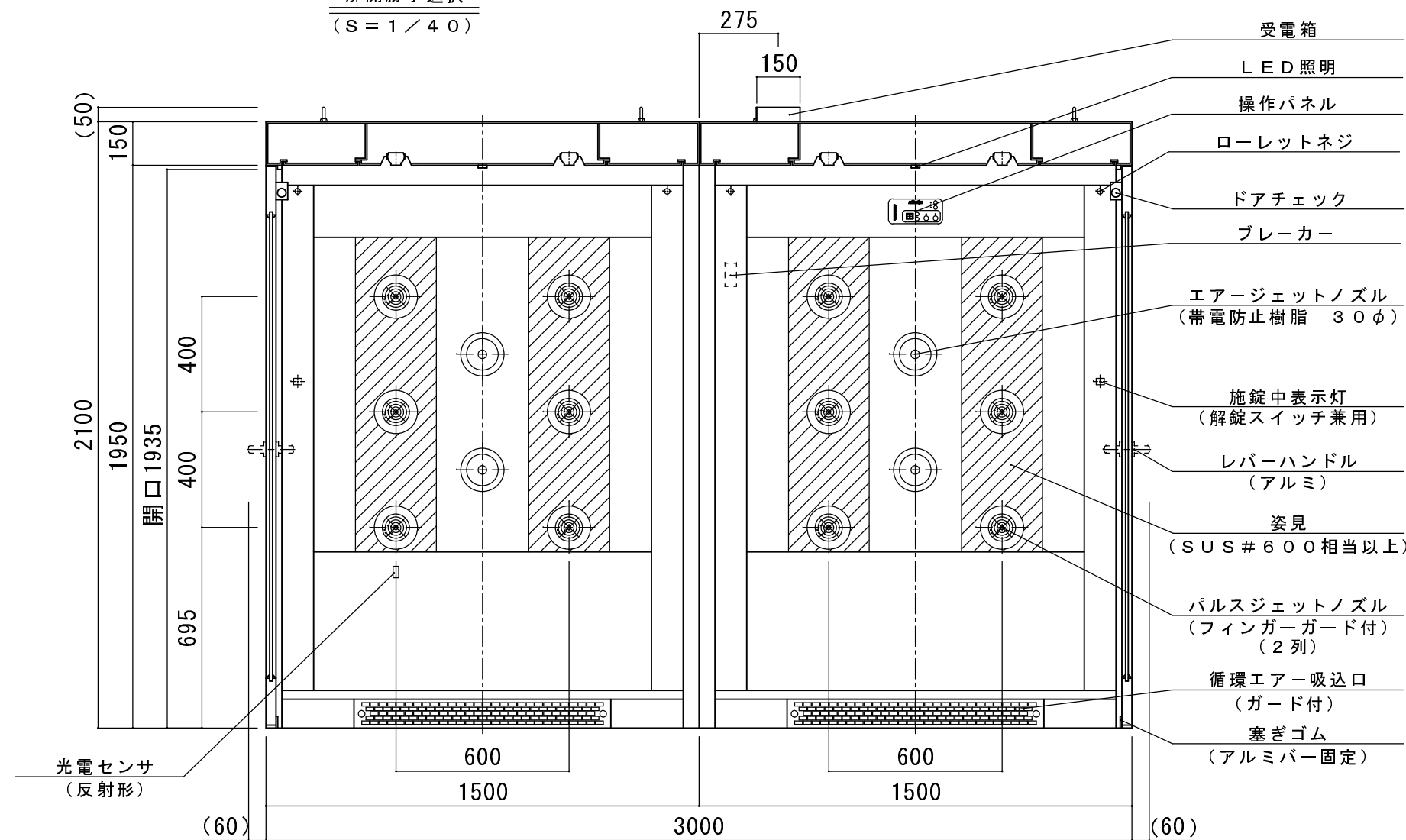
A-A' 断面
