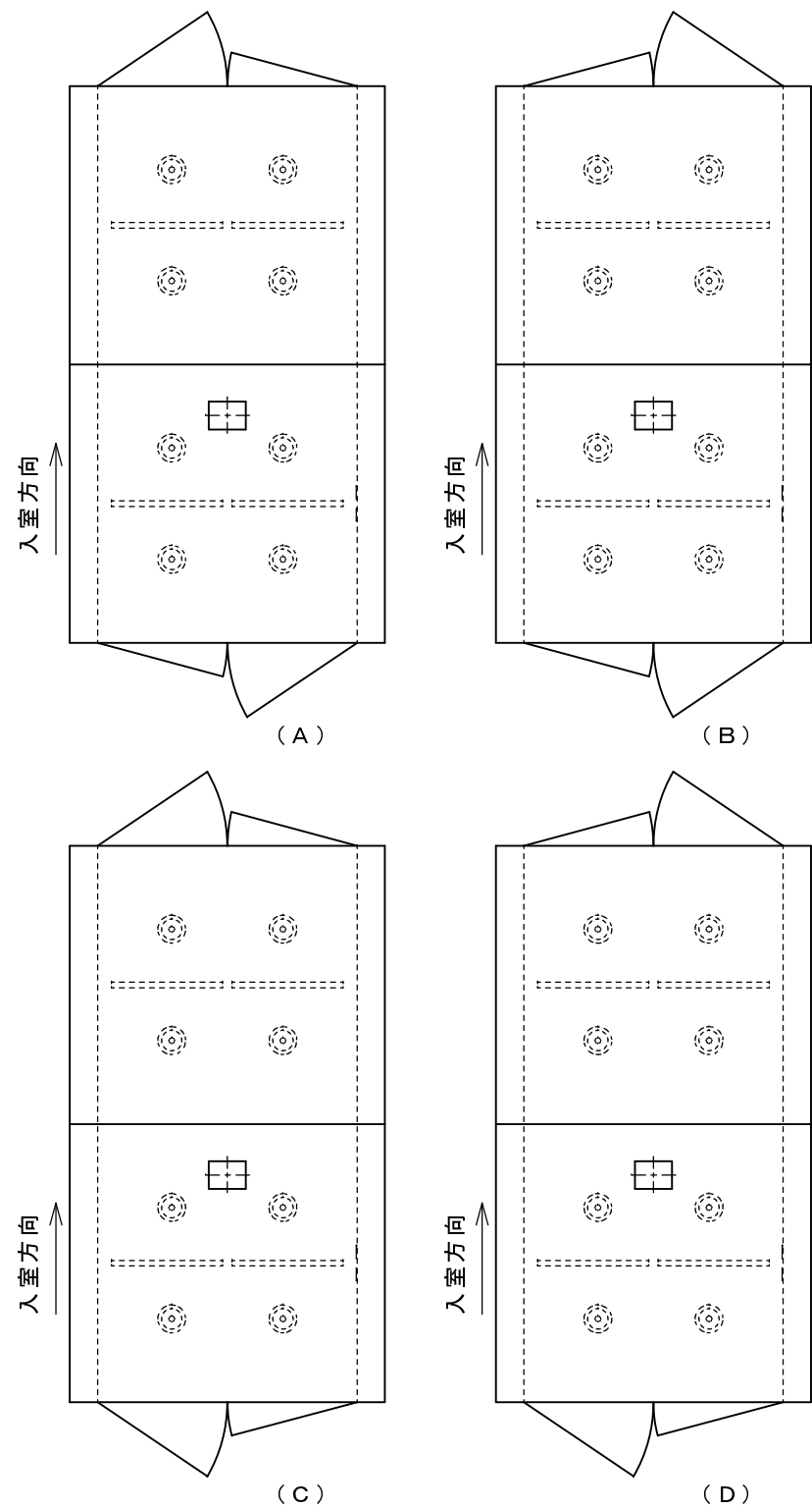
扉開勝手選択 (S=1/40)
