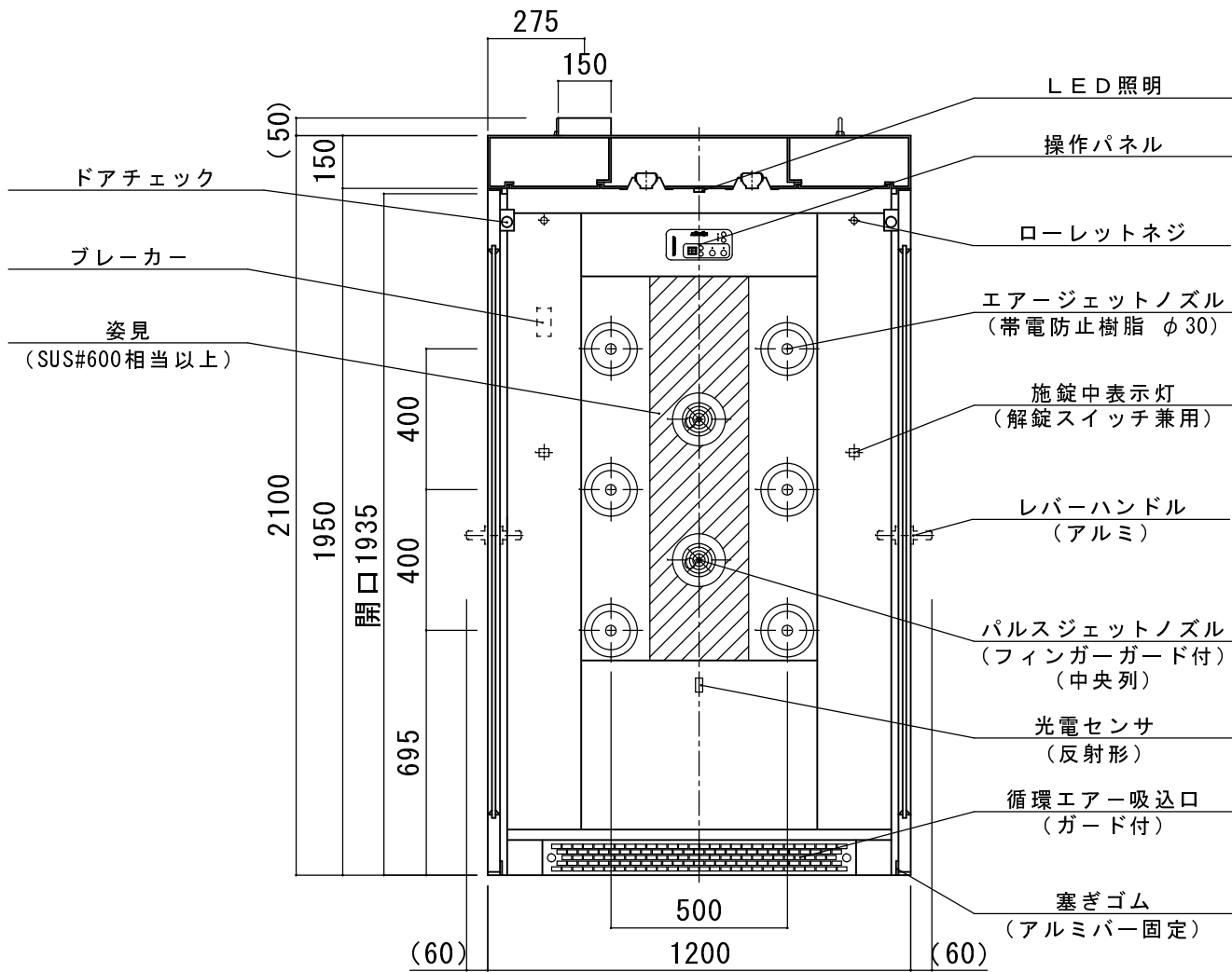
A-A' 断面
