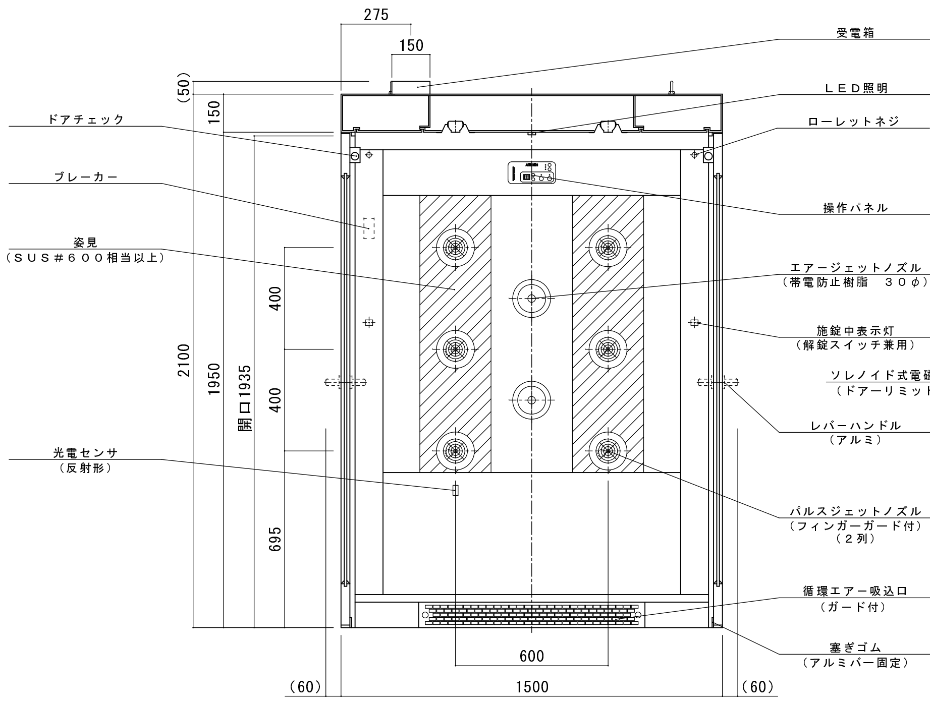
A-A'断面
