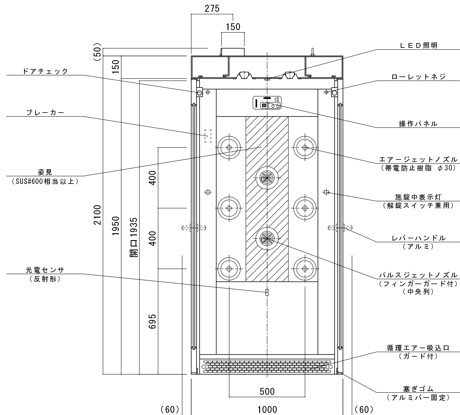
A-A' 断面
