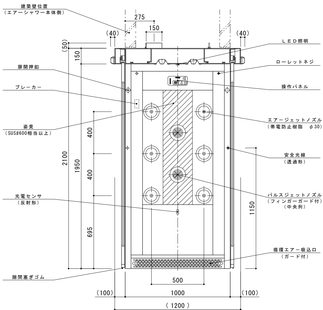
A-A' 断面
