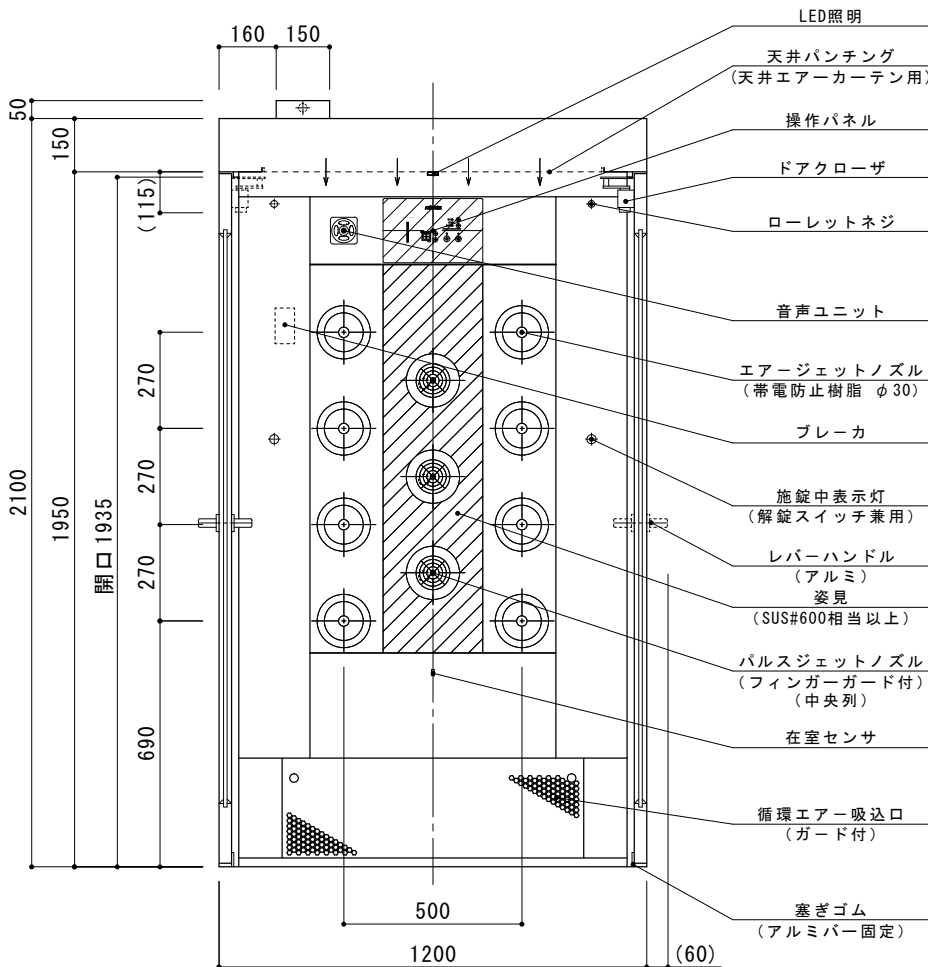
A-A' 断面
