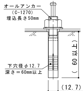
アンカー施工図 (S=1/2)
