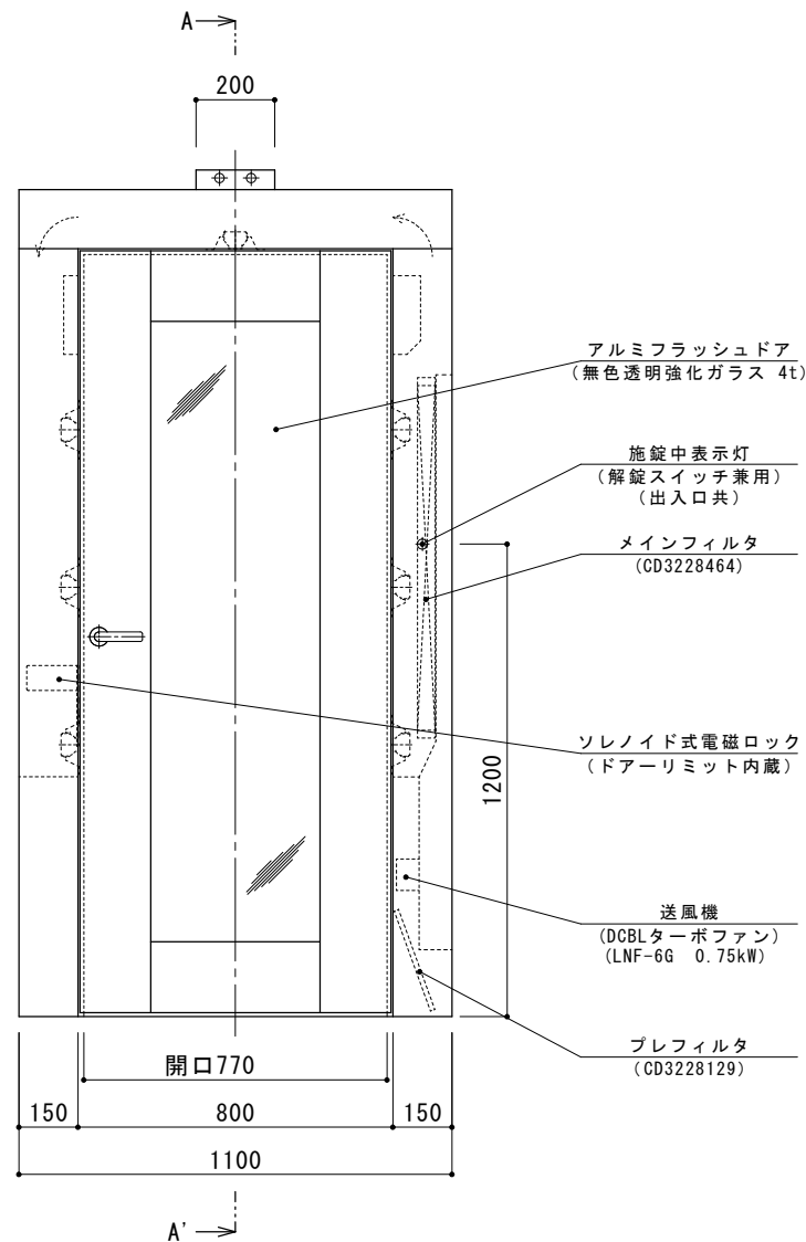
扉開勝手仕様 (S=1/40)
