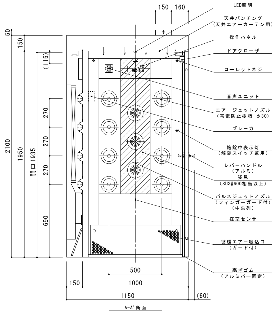
A-A'断面
