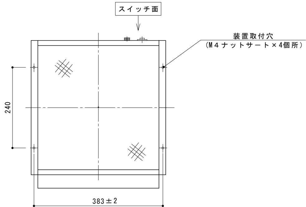
A 矢視図 (S=1/7)
