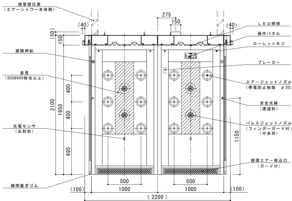
A-A' 断面
