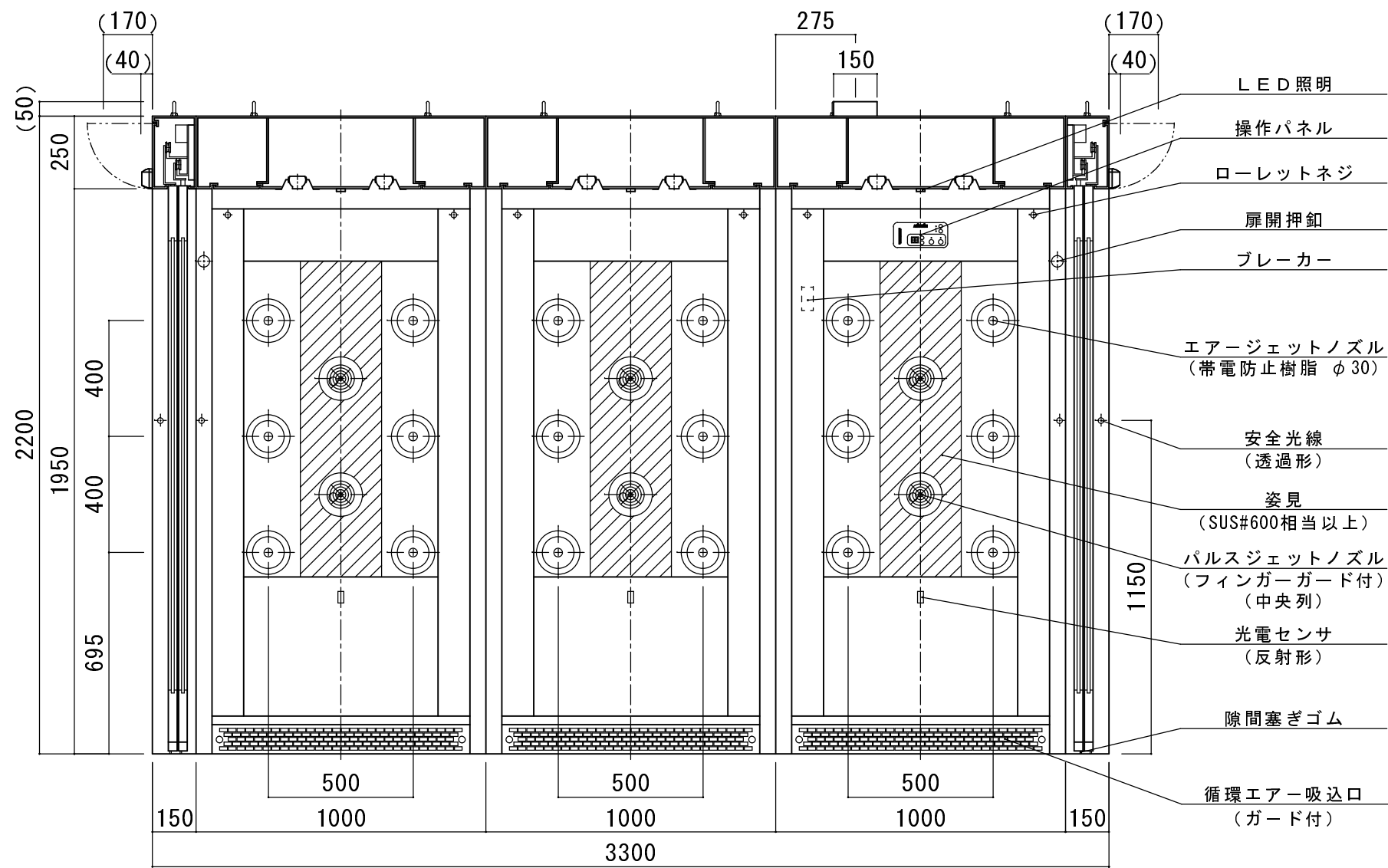
A-A' 断面
