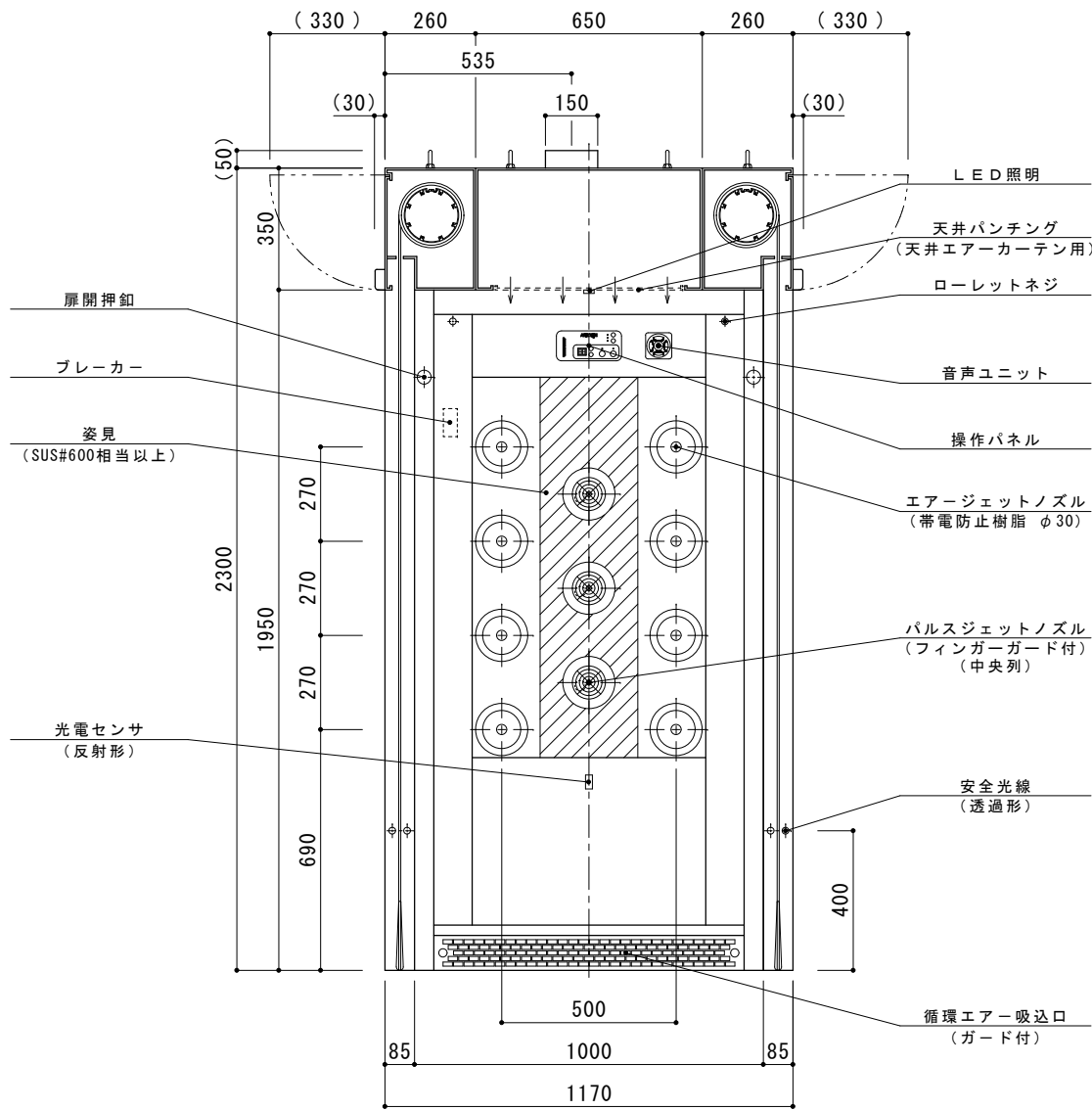
A-A' 断面
