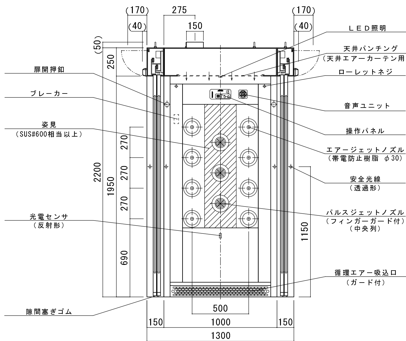
A-A' 断面
