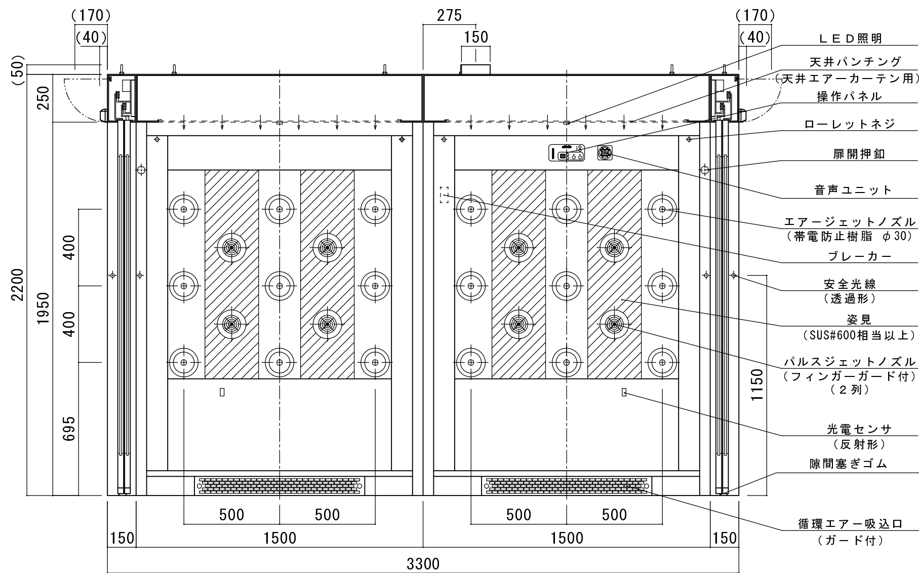
A-A' 断面
