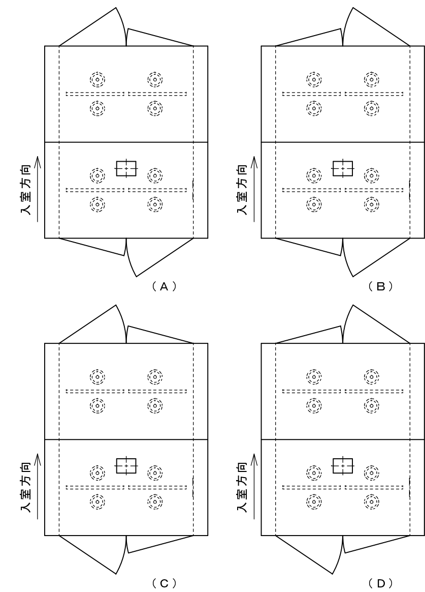
扉開勝手選択 (S=1/40)
